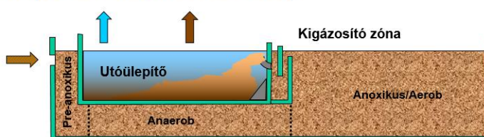
2. ábra – A biológiai tisztítás fizikai kialakítása
